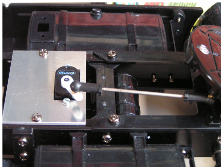
Abbildung 10: Servo für die Sattelpuplung
