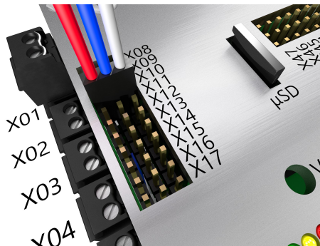
Abbildung 12: Schaltausgänge
