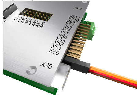
Abbildung 5: Belegung der Servokabel Abbildung 6: Orientierung der Empfänger-Servokabel
