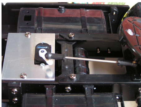
Abbildung 9: Servo für die Sattelpkupplung
