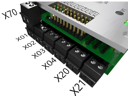
Abbildung 10: Motorsteckverbinder
