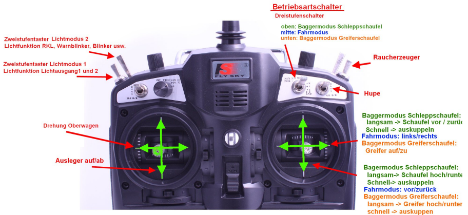
Abbildung 1: Beispielhafte Senderbelegung
