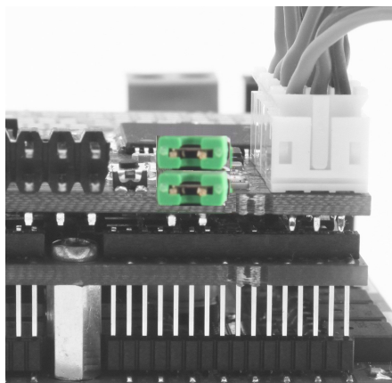
Abbildung 6: BEC Spannung nicht wei- terleiten
