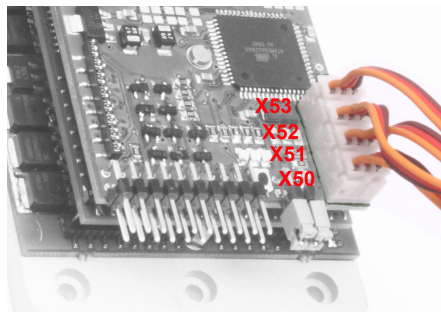
Abbildung 5: Belegung der Servoleitungen
