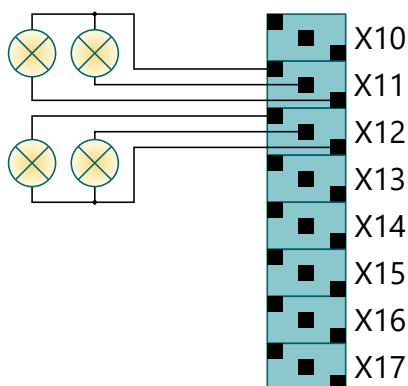
Abbildung 18: Rundumlichtverdrahtung
