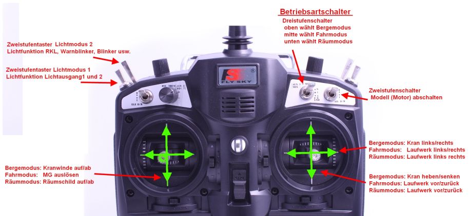
Abbildung 1: Beispielhafte Senderbelegung
