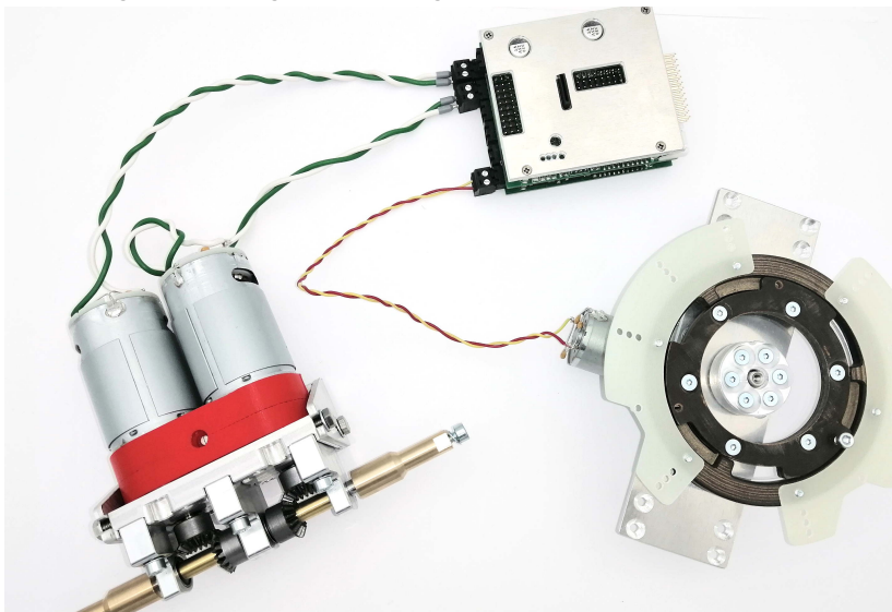
Abbildung 11: Wird unser Getriebe vorne in das Fahrzeug gebaut, wird der linke Motor (in Fahrrichtung) an X01 angeschlossen. Weiße Leitung an X01+, grüne Leitung an X01-. Der rechte Motor (in Fahrrichtung) wird an X02 angeschlossen. Weiße Leitung an X02+, grüne Leitung an X02-.
