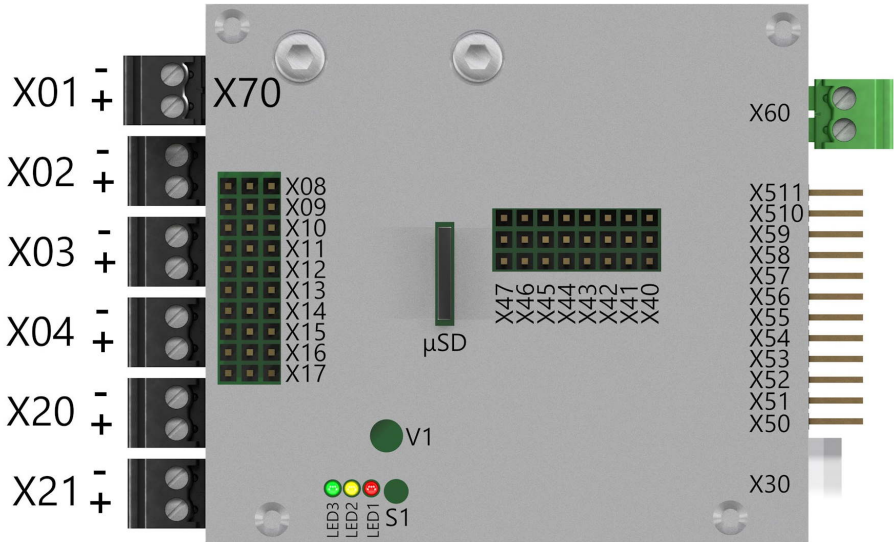
Abbildung 1: Übersicht der Anschlussklemmen
