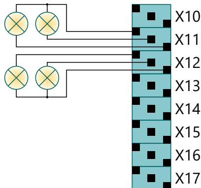
Abbildung 20: Rundumlichtverdrahtung
