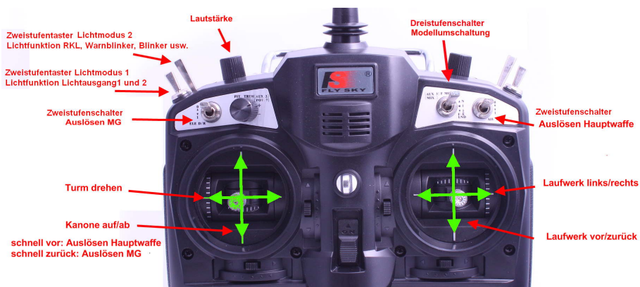
Abbildung 1: Beispielhafte Senderbelegung
