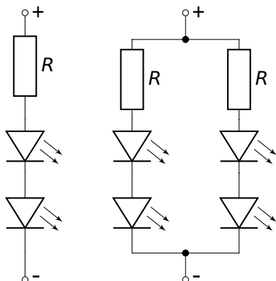
Abbildung 22: Vorwiderstand mehrerer LEDs
