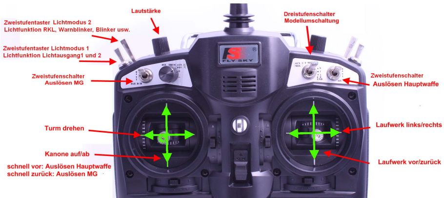
Abbildung 1: Beispielhafte Senderbelegung
