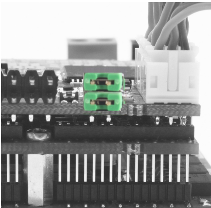
Abbildung 7: BEC Spannung nicht weiterleiten
