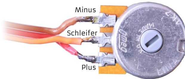
Abbildung 6: Anschluss des Potentiometers
