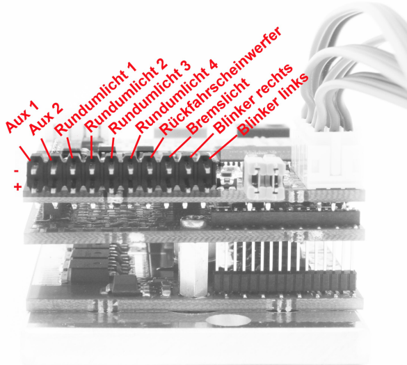
Abbildung 9: Belegung der Lichtausgänge
