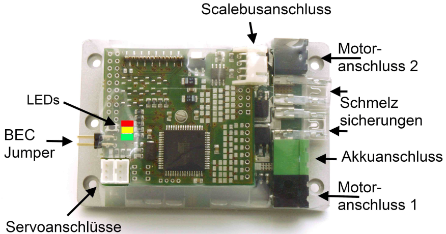
Abbildung 2: Übersicht der Anschlüsse
