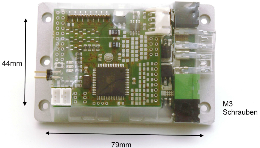
Abbildung 1: Befestigungsbohrungen
