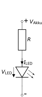
Abbildung 20: Vorwiderstand einer LED
