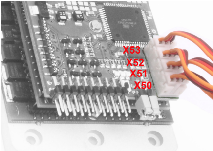
Abbildung 3: Belegung der Servostecker
