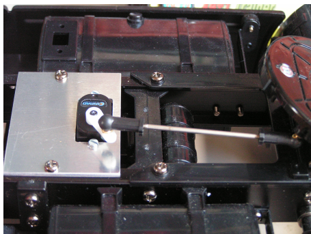
Abbildung 9: Servo für die Sattelkupplung
