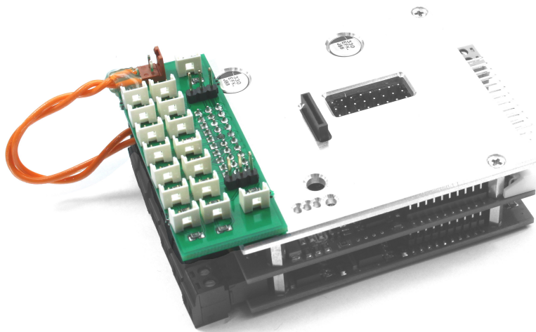
Abbildung 1: Funktion der Stecker am Adapter
