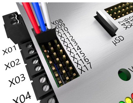
Abbildung 11: Schaltausgänge
