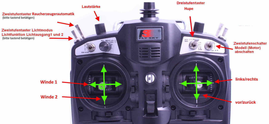
Abbildung 1: Beispielhafte Senderbelegung
