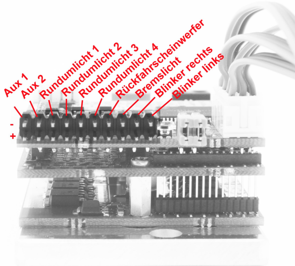
Figure 8: Belegung der Lichtausgänge
