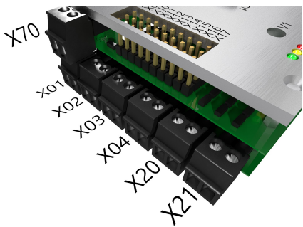
Abbildung 10: Motorsteckverbinder
