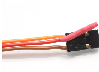
Abbildung 5: entfernte und isolierte + Zuleitung im Servostecker
