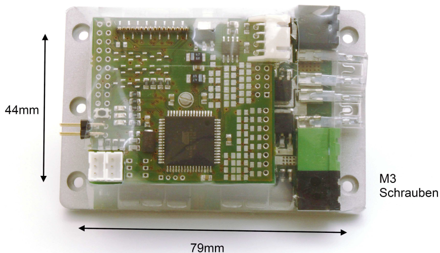
Abbildung 1: Befestigungsbohrungen
