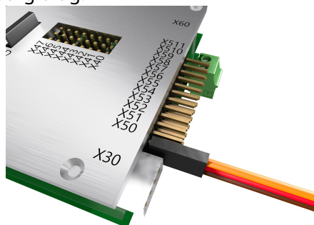
Abbildung 8: Orientierung der Empfänger-Servokabel
