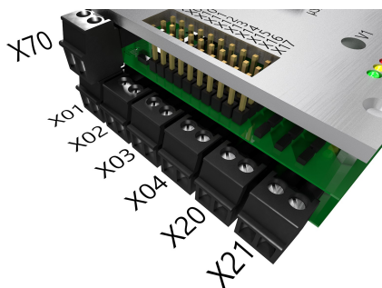
Abbildung 12: Motorsteckverbinder
