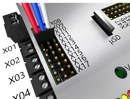
Abbildung 15: Schaltausgänge
