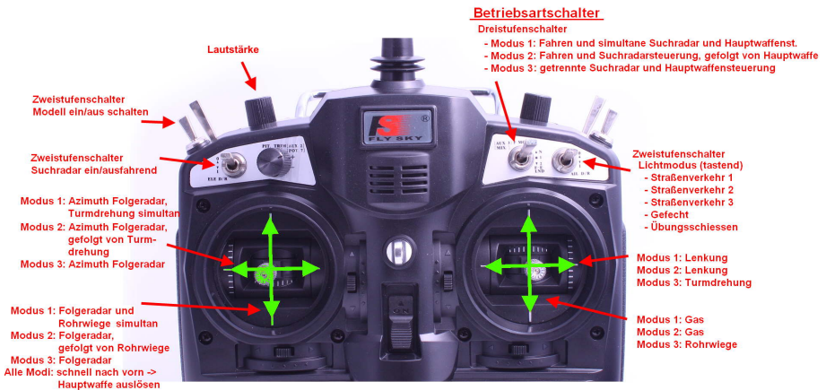
Abbildung 1: Beispielhafte Senderbelegung
