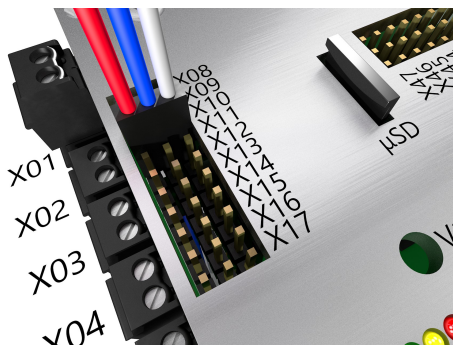
Abbildung 13: Schaltausgänge
