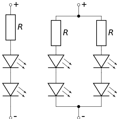
Abbildung 20: Vorwiderstand mehrerer LEDs
