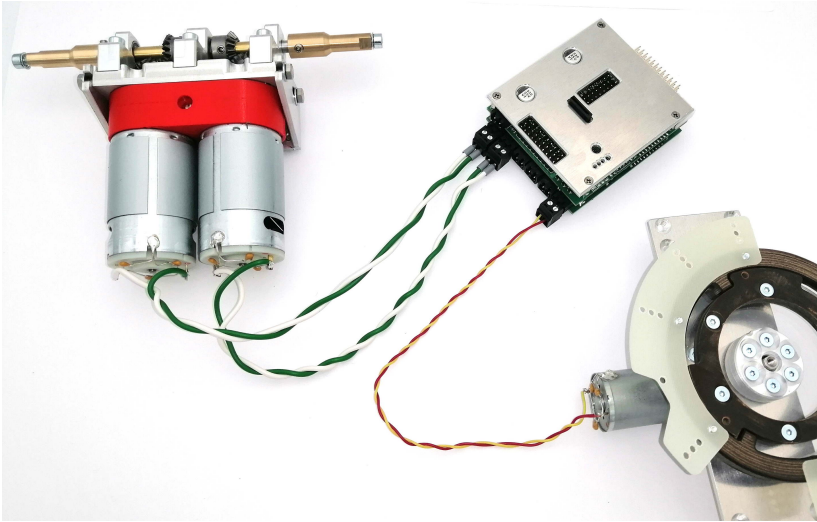
Abbildung 11: Wird unser Getriebe vorne in das Fahrzeug gebaut, wird der linke Motor (in Fahrrichtung) an X01 angeschlossen. Weiße Leitung an X01+, grüne Leitung an X01-. Der rechte Motor (in Fahrrichtung) wird an X02 angeschlossen. Weiße Leitung an X02+, grüne Leitung an X02-.
