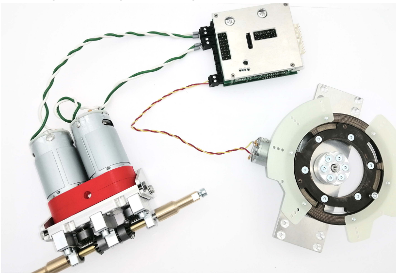
Abbildung 11: Wird unser Getriebe vorne in das Fahrzeug gebaut, wird der linke Motor (in Fahrrichtung) an X01 angeschlossen. Weiße Leitung an X01+, grüne Leitung an X01-. Der rechte Motor (in Fahrrichtung) wird an X02 angeschlossen. Weiße Leitung an X02+, grüne Leitung an X02-.
