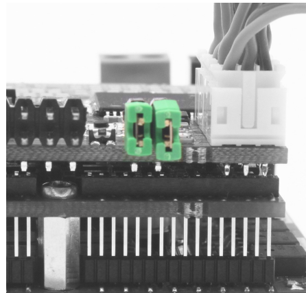
Abbildung 8: BEC Spannung weiterleiten
