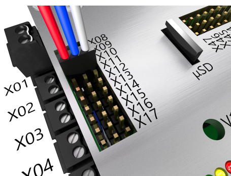
Abbildung 11: Schaltausgänge
