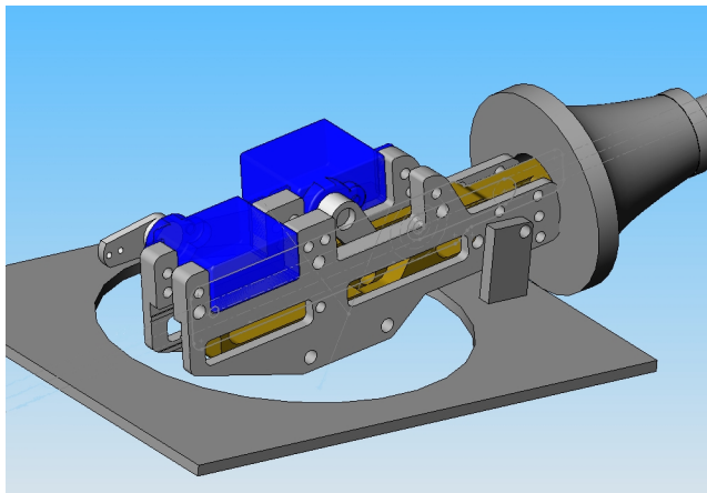
Abbildung 9: Beispiel einer Rohranhebe und Rückzugseinheit mit Servos
