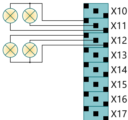
Abbildung 20: Rundumlichtverdrahtung
