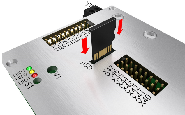
Abbildung 21: Position der \mu SD Karte
