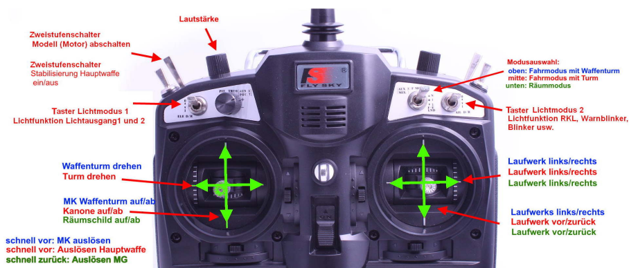
Abbildung 1: Beispielhafte Senderbelegung
