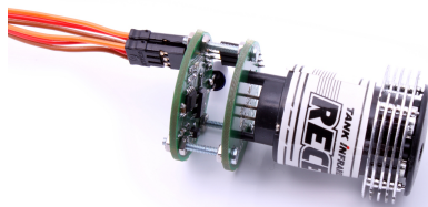
Abbildung 19: TVC-BU12
