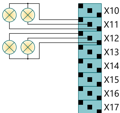
Abbildung 23: Rundumlichtverdrahtung
