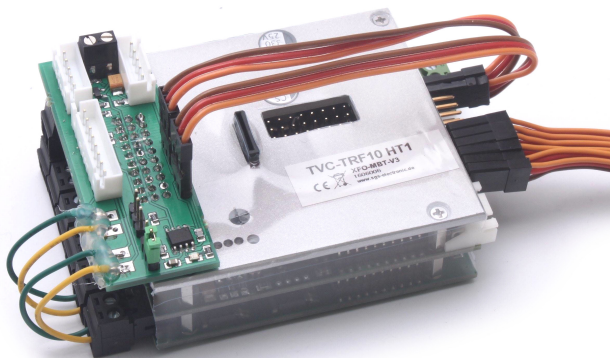
Abbildung 20: TVC-HRF-AD3 montiert auf dem FO Module
