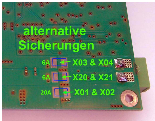
Abbildung 22: Lage der Sicherungen für die Motoren
