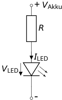
Abbildung 24: Vorwiderstand einer LED
