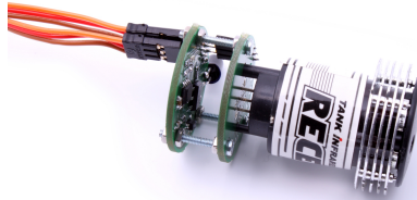
Abbildung 19: TVC-BU12
